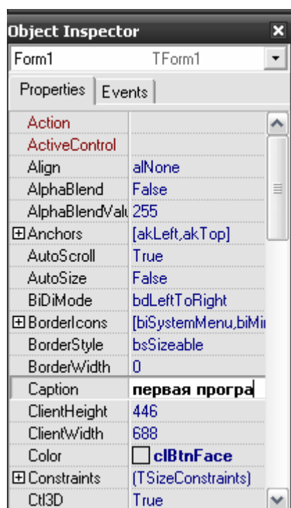
Рис.1.3. Изменение заголовка окна программы
