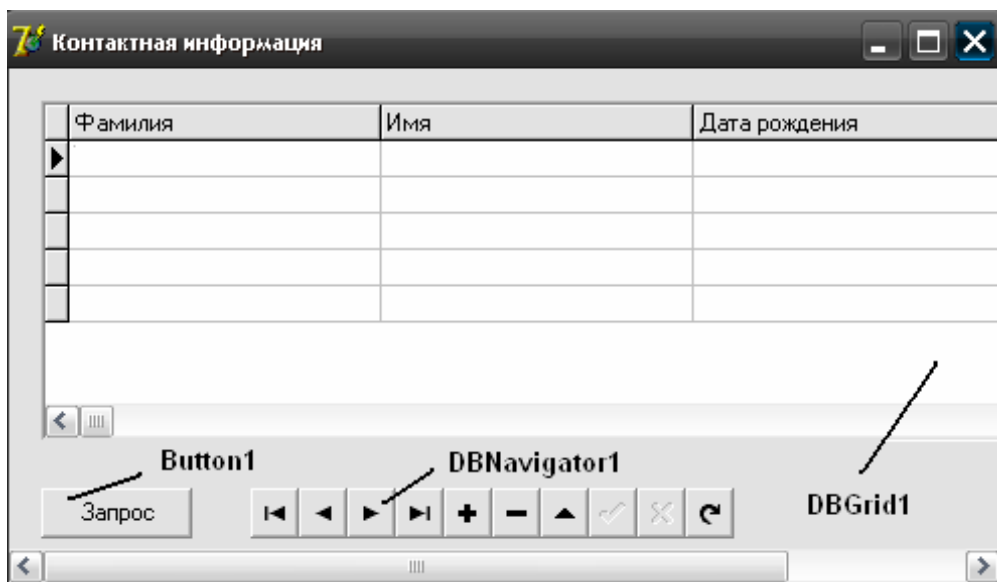
Рис. 6.6. Программа управления базой данных с просмотром в режиме таблицы
